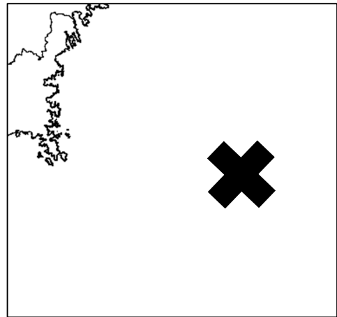
資料イ 震源地
