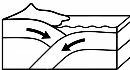
資料ウ 地震発生のメカニズム
