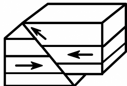
資料エ 地震発生のメカニズム
