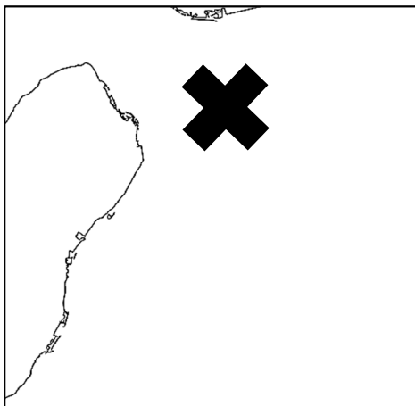
資料ア 震源地
